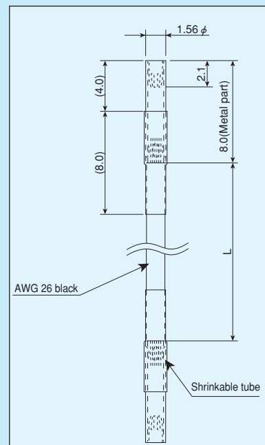
PRW-0.7-□
