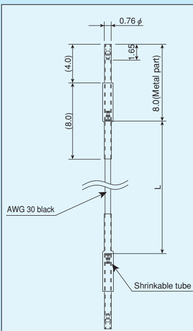
PRW-0.3-□
