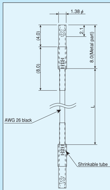
PRW-0.5-□
